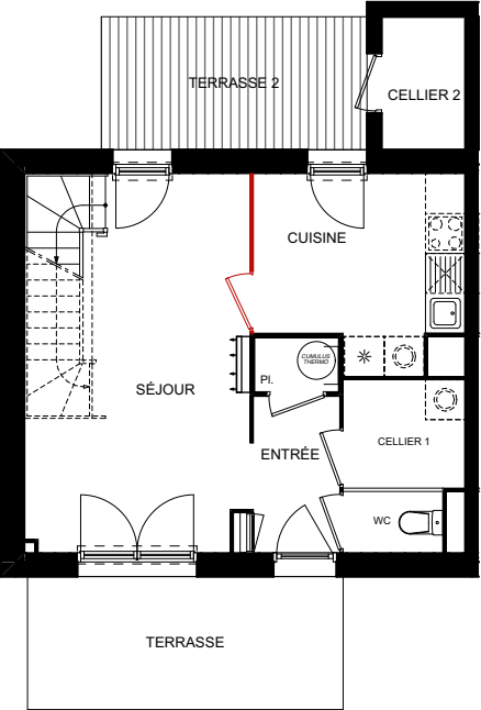
RDC - VARIANTE 1
