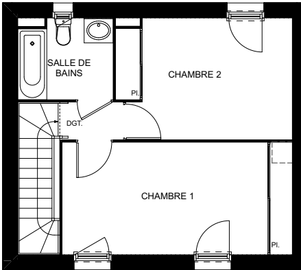
ÉTAGE - BASE
