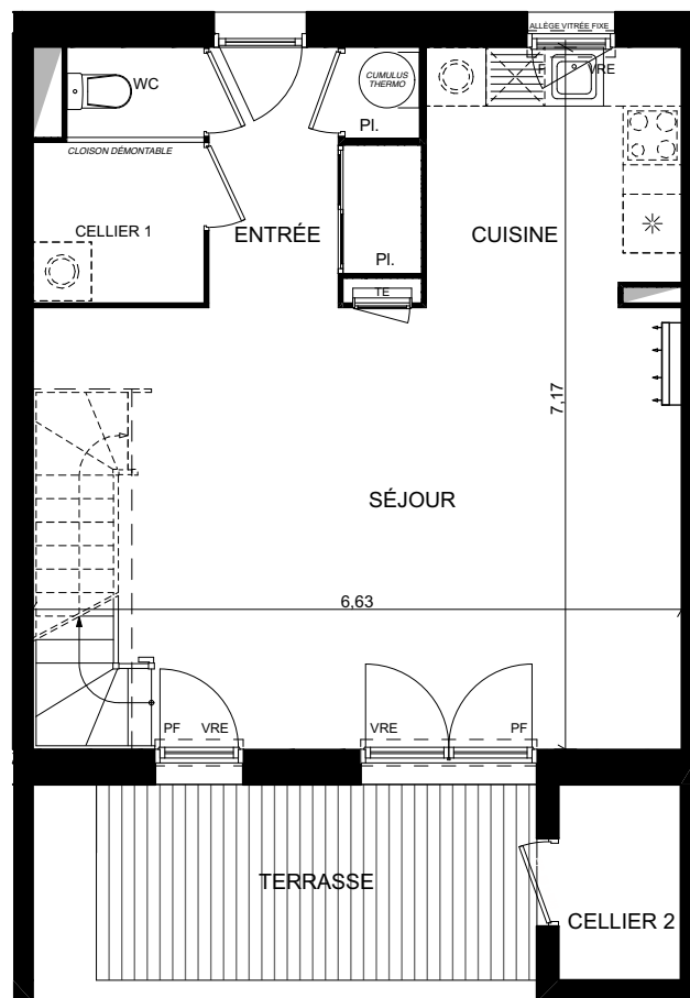
REZ DE CHAUSSEE
