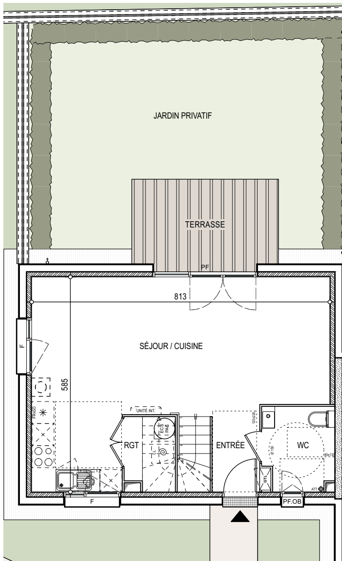
REZ-DE-CHAUSSÉE
