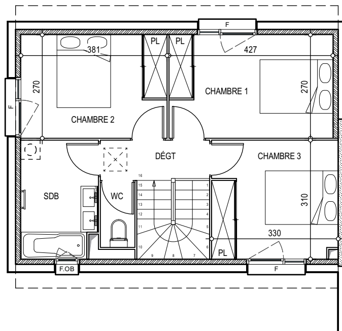
ÉTAGE
