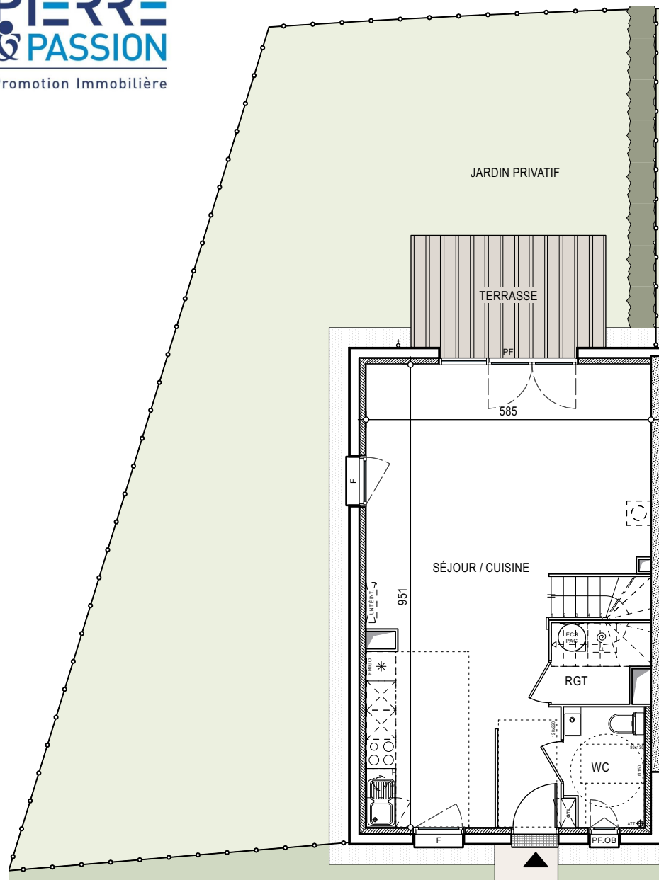
REZ-DE-CHAUSSÉE
