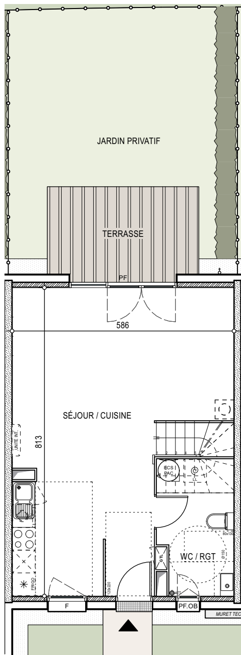
REZ-DE-CHAUSSÉE
