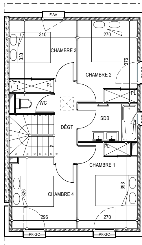
ÉTAGE
