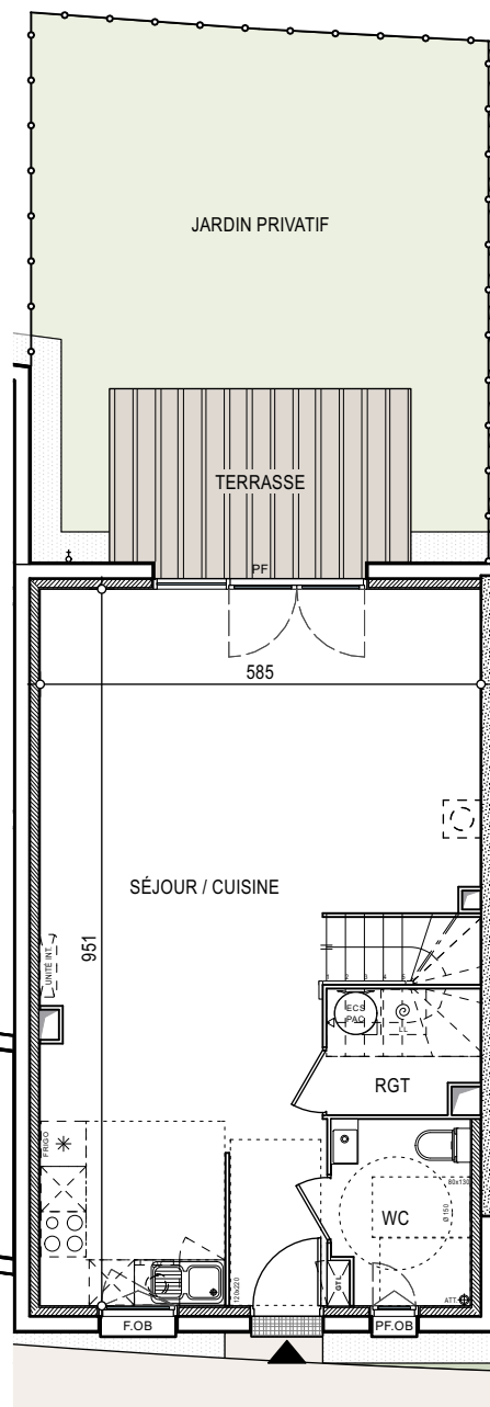
REZ-DE-CHAUSSÉE
