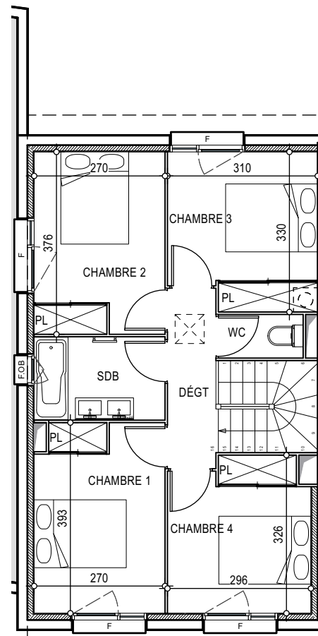
ÉTAGE
