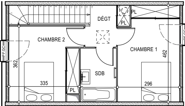
ÉTAGE
